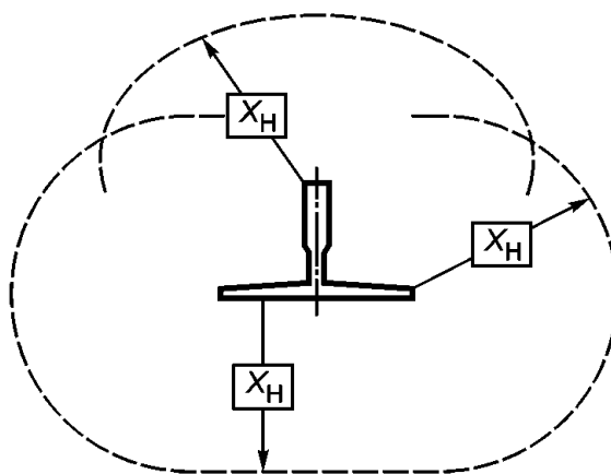
Рисунок 6 - Горизонтальное расстояние X_H вокруг направляющей
