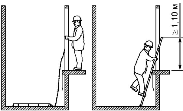
Тип 3а - Передвижная лестница прямка
