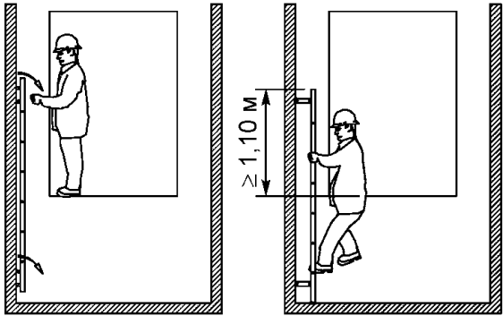
Тип 2а - Выдвижная лестница прямка
