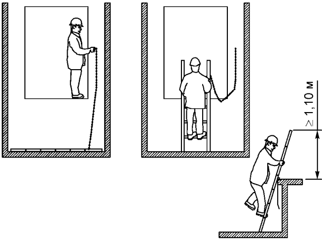
Тип 3б - Передвижная лестница прямка
