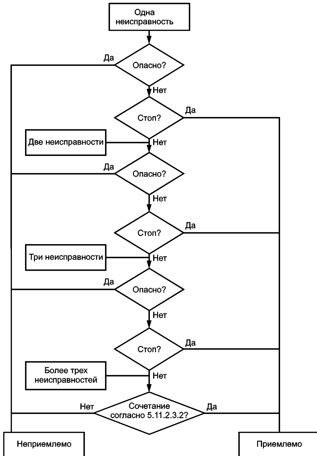
Рисунок 25 - Блок-схема оценки цепи безопасности
