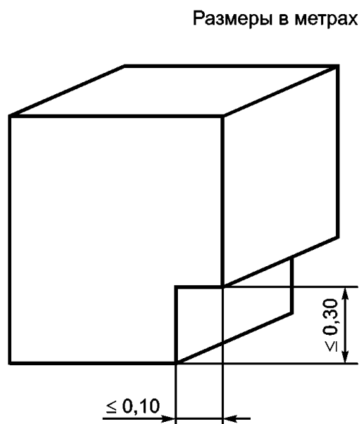
Рисунок 4 - Максимальные уменьшения пространств безопасности для персонала
