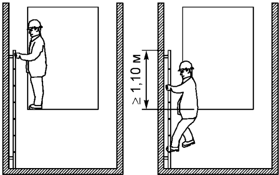
Тип 1 - Фиксированная лестница прямка
