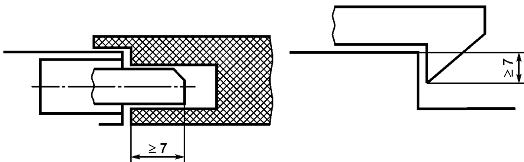
Рисунок 12 - Примеры запирающих элементов
