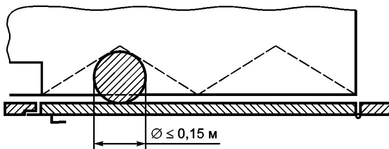
Рисунок 8 - Распашная дверь шахты и складная дверь кабины
